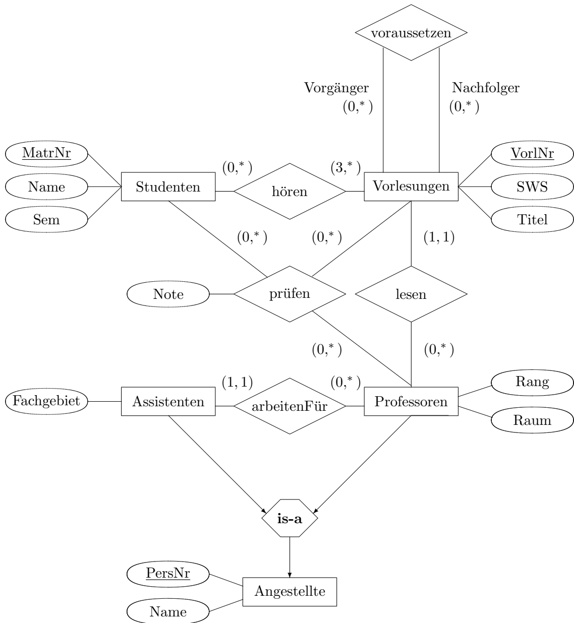
Abbildung 1: Das Beispielschema der Universität mit (min,max) -Angabe und einer Generalisierung
